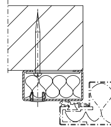
Einbau in Mauerwerk: (Aufschraubrahmen)
