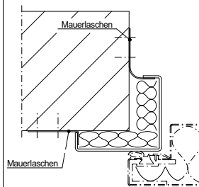
Einbau in Mauerwerk: (Aufschraubrahmen)
