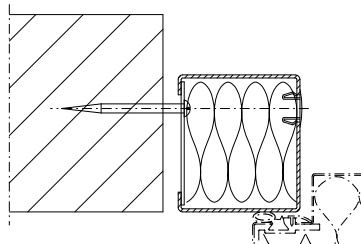
Einbau in Mauerwerk: (Durchschraubrahmen)
