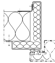
Einbau in Mauerwerk: (Winkelrahmen)
