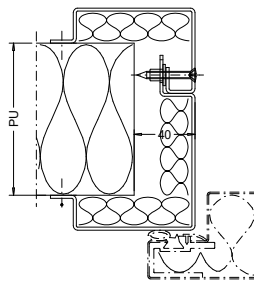
Einbau in Mauerwerk: (Durchschraubrahmen)
